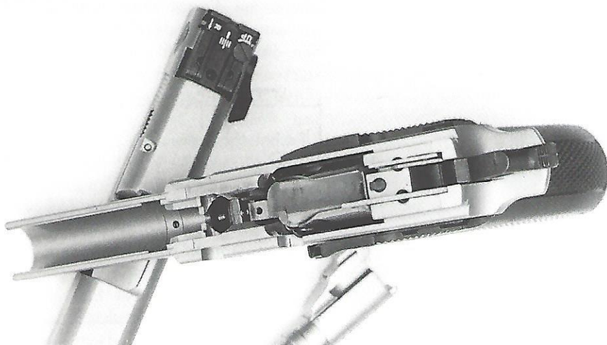
Het binnenwerk. De slede wordt niet over de gehele lengte geleid, maar via relatief korte rails voor en achter de magazijnopening. Hierdoor is een strakkere passing mogelijk
